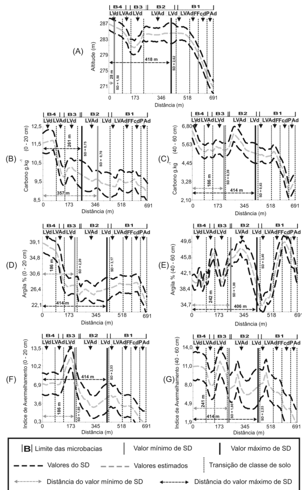
Figura 2 - Valores estimados por krigagem ordinária da altitude (A), carbono orgânico (B e C), argila (D e E) e índice de avermelhamento (F e G), nas profundidades de 0-20 e 40-60 cm, ao longo do transecto na direção oeste-leste.
